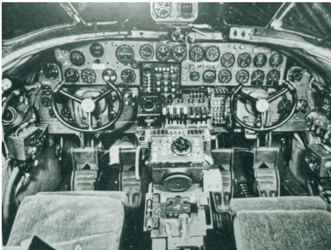
B-24-es bombázó pilótakabin műszerfala
